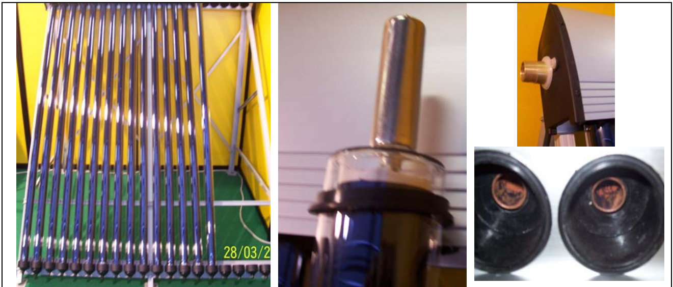
Il pannello ed il particolare dell'Heat Pipe e alcuni dettagli
